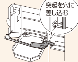
支え部品を取り付ける
